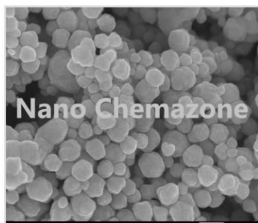
Bismuth Nanopowder
